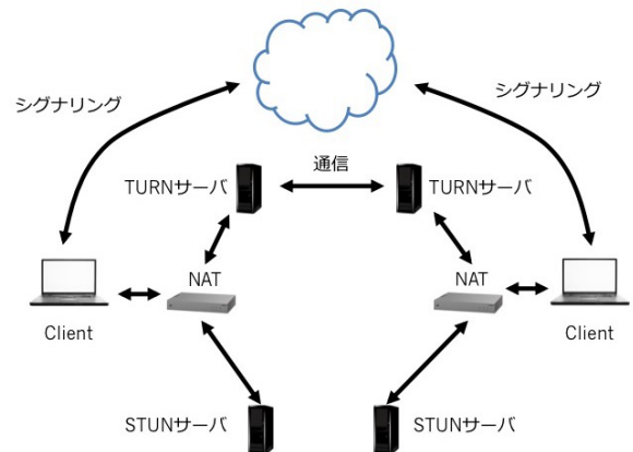
図 5 TURN によるサーバ経由通信
