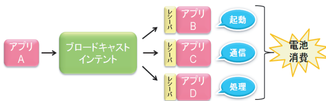
図 2 アプリケーション、ブロードキャストインテント、電池消費の因果関係
