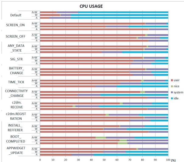
図 3 CPU 使用率
