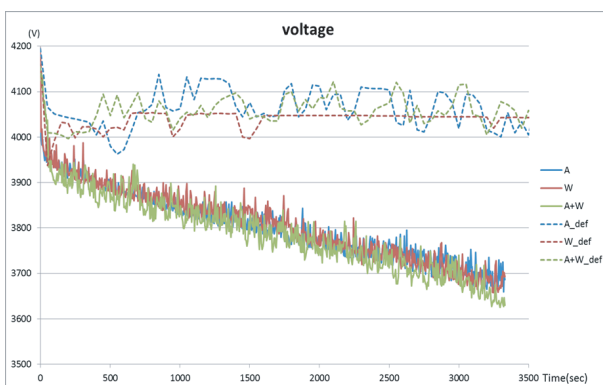
図6 電圧変動
