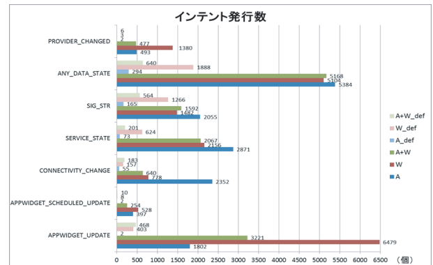
図7 logcatで取得したIntentの一部
