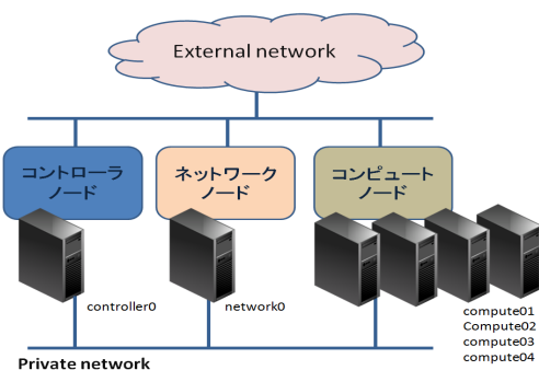
図 4: OpenStack によるクラウド構築
