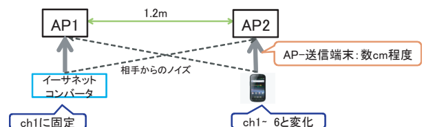
図 6 無線 LAN の配置
