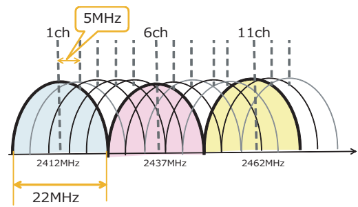
図 1 無線 LAN 周波数
