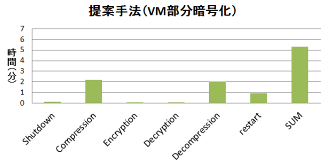
図 7 VM の部分を暗号化する場合の固定時間
