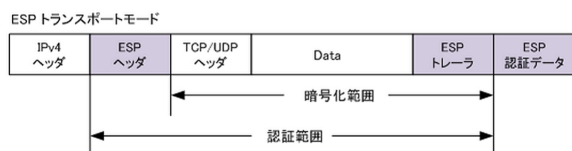
図 4 トランスポートモードにおける EPS カプセル化パケット
