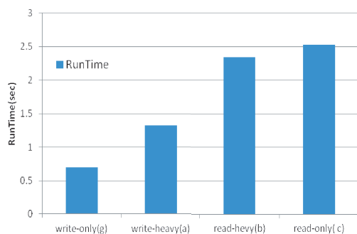
図 1: 各種ワークロードの実行時間
