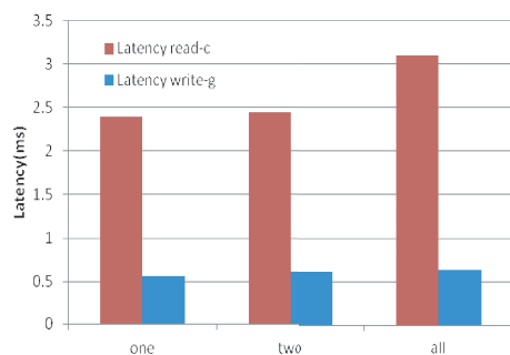
図 2: ワークロード c, g の読み出し，書き込み処理の際に生じる遅延
