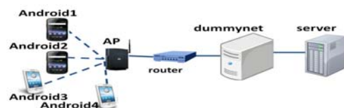
図 4: ヘテロ端末環境
