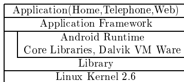
図 1: Android のアーキテクチャ
