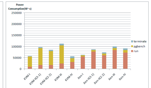
図 15 評価 2:消費電力量
