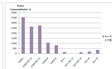
図 22 評価 5:消費電力量の差
