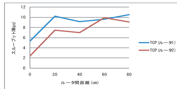
図 7 TCP—TCP の相互干渉 (1 台通信時)
