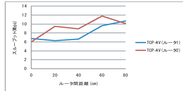
図 11 TCP-AV—TCP-AV の相互干渉 (1 台通信時)
