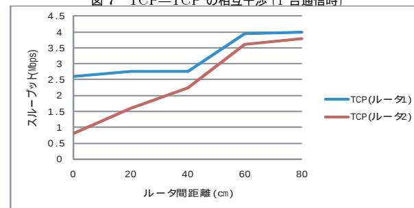
図 8 TCP—TCP の相互干渉 (5 台通信時)
