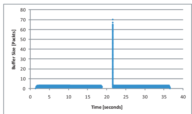
図 8 パケットロスが起こった際の受信側バッファへ溜まったパケット量
