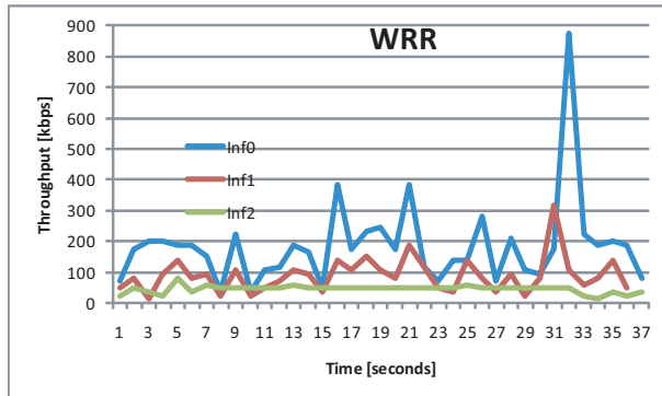
図 4 WRR を用いた場合のスループット
