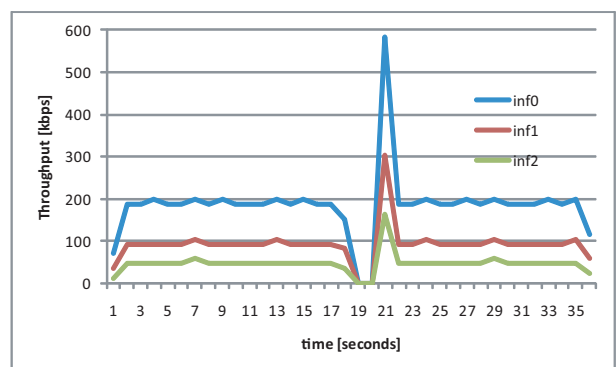
図 7 パケットロスが起こった際の EDPF のスループット
