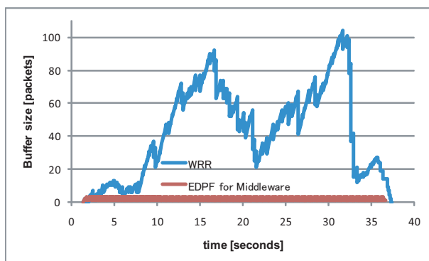
図 5 受信側バッファへ溜まったパケット量
