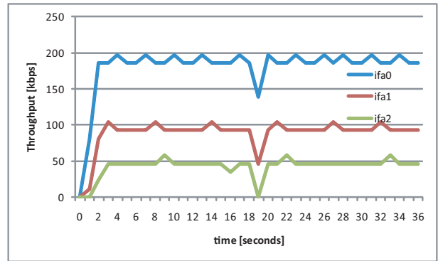
図 6 ネットワーク層での制御でパケットロスが起こった際のスループット
