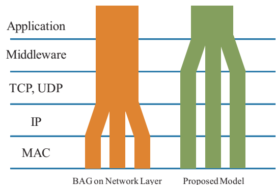
図 1 提案手法
