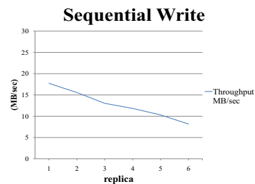
図 6 Write スループット Fig. 6 Write throughput
