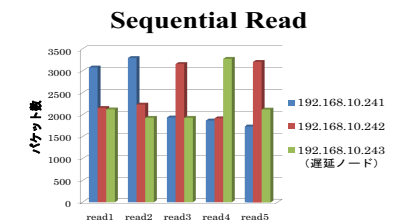
図 21 read 実行時のパケット数 Fig. 21 Exchanged Packets under Read Program
