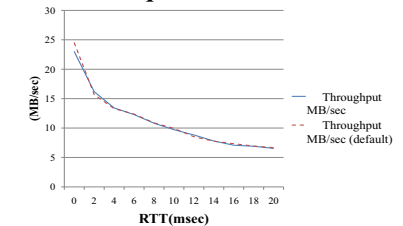
図 17 Read スループット Fig. 17 Read throughput
