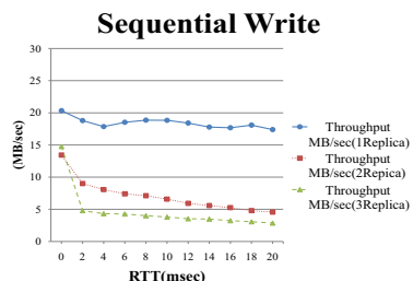
図 9 Write スループット Fig. 9 Write throughput
