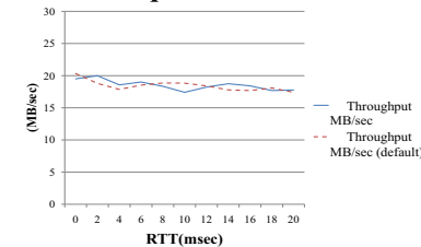
図 16 Write スループット Fig. 16 Write throughput
