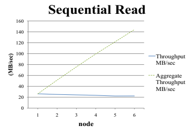
図 5 Read スループット Fig. 5 Read throughput
