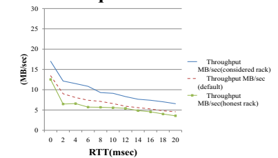
図 15 Read スループット Fig. 15 Read throughput
