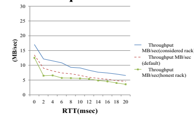
図 14 Write スループット Fig. 14 Write throughput
