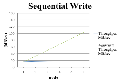
図 4 Write スループット Fig. 4 Write throughput
