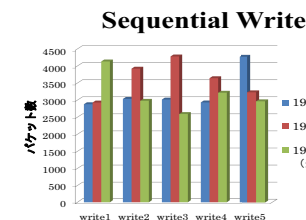
図 20 write 実行時のパケット数 Fig. 20 Exchanged Packets under Write Program
