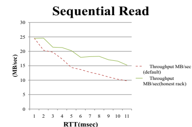
図 13 Read スループット Fig. 13 Read throughput
