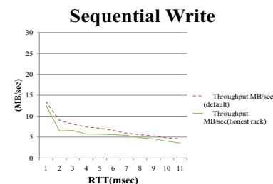
図 12 Write スループット Fig. 12 Write throughput
