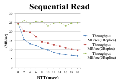
図 10 Read スループット Fig. 10 Read throughput
