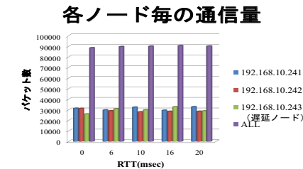
図 19 各ノードとの通信量 Fig. 19 Number of Exchanged Packets among Namenode and each Datanode
