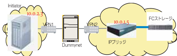
図 1: VPN 遠隔接続環境
