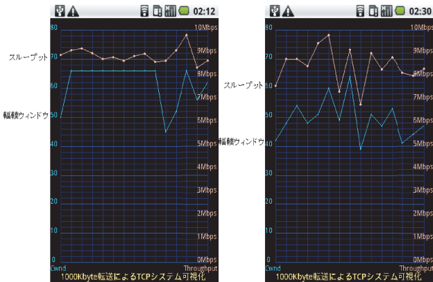
図 3: 同一無線 LAN 内に Android 端末 1 台のみの通信状況 図 4: 同一無線 LAN 内に Android 端末 4 台の通信状況
