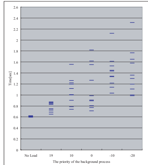
図 15 宛先ノード C からデータ配信し全端末においてデータ受信及び再生した場合
