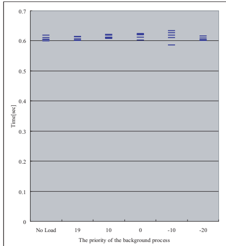
図 7 中継ノード B からデータ配信し同一端末でデータ受信及び再生した場合
