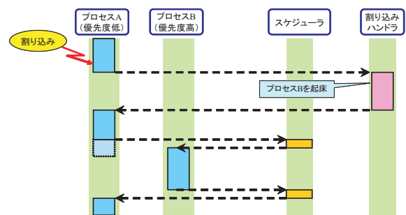
図3 プリエンプティブな場合の割り込み処理
