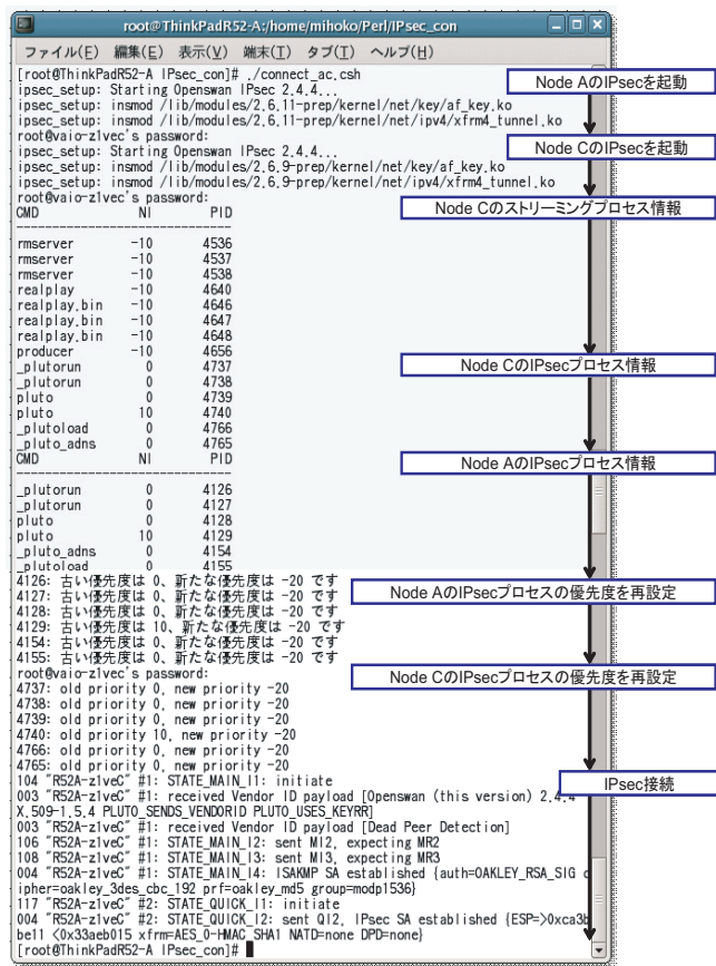
図 18 IPsec 自動接続プログラムの実行例
