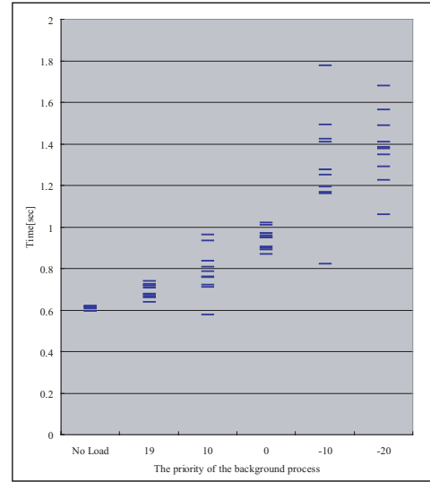
図 14 宛先ノード C からデータ配信し中継ノード B でデータ受信及び再生した場合
