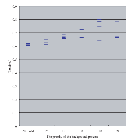
図 9 中継ノード B からデータ配信し宛先ノード C でデータ受信及び再生した場合
