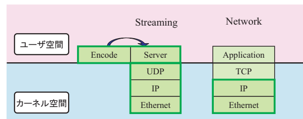
図 11 中継ノード B における処理
