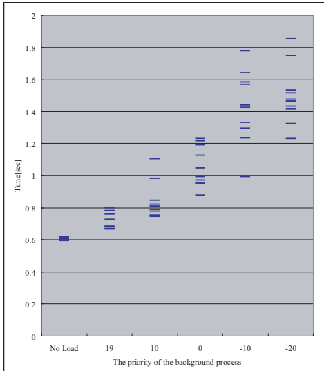
図 13 宛先ノード C からデータ配信し送信元ノード A でデータ受信及び再生した場合
