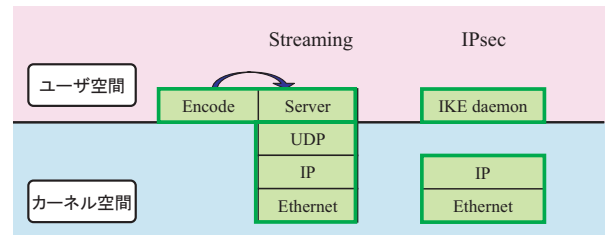
図 16 宛先ノード C における処理
