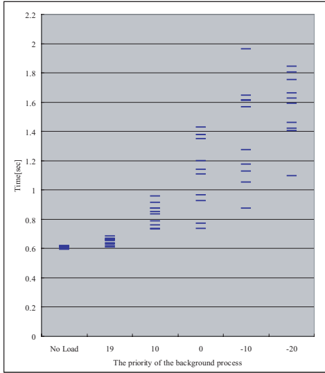
図 12 宛先ノード C からデータ配信し宛先ノード C でデータ受信及び再生した場合
