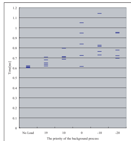
図 10 中継ノード B からデータ配信し全端末においてデータ受信及び再生した場合
