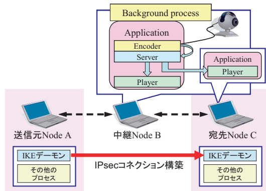
図 6 マルチホップ通信
