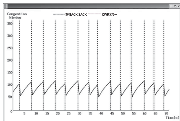
図 5: 輻輳ウィンドウの変化 (VPN あり)
