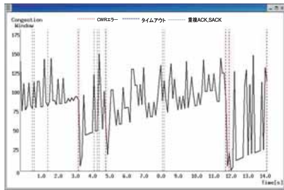
図 14: 輻輳ウィンドウの変化（VPN なし）
