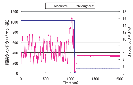
図 17: スループットの変化 (VPN なし)
