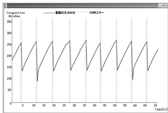
図 4: 輻輳ウィンドウの変化 (VPN なし)
