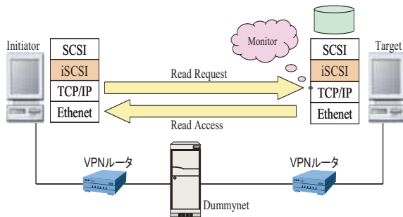
図 3: 1 対 1 通信時の実験環境
