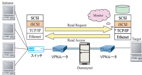
図 13: 複数台 Initiator の実験環境
