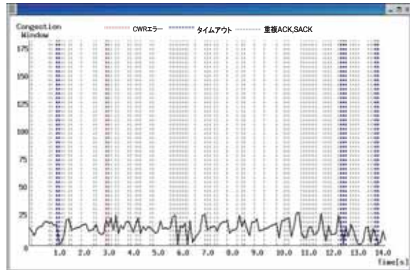
図 15: 輻輳ウィンドウの変化（VPN あり）
