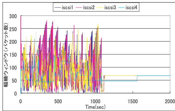
図 16: 輻輳ウィンドウの変化 (VPN なし)
