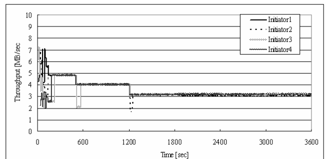
図4 提案手法Iを用いた場合のスループット時間変化 Fig.4 Throughput using the Proposed Method(I)
