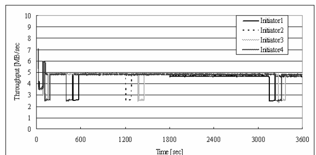
図6 提案手法 II を用いた場合のスループット時間変化 Fig.6 Throughput using the Proposed Method(II)
