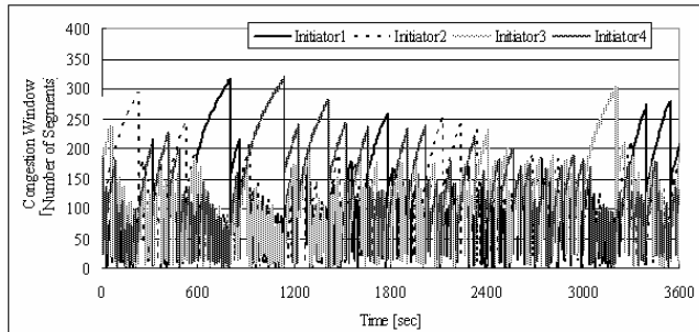
図1 提案手法を用いない場合の輻輳ウィンドウ時間変化 Fig.1 Congestion Window not using the Proposed Method
