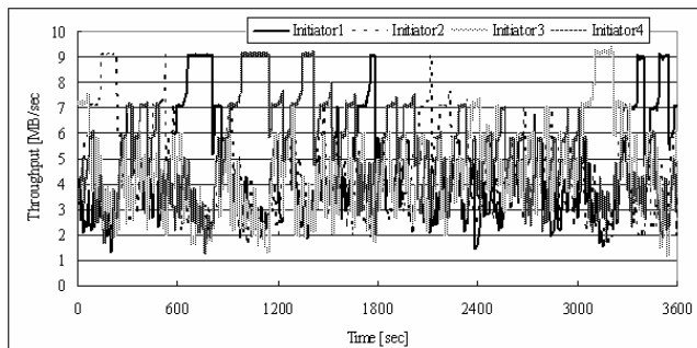
図2 提案手法を用いない場合のスループット時間変化 Fig.2 Throughput not using the Proposed Method
