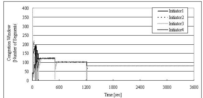
図3 提案手法Iを用いた場合の輻輳ウィンドウ時間変化 Fig.3 Congestion Window using the Proposed Method(I)
