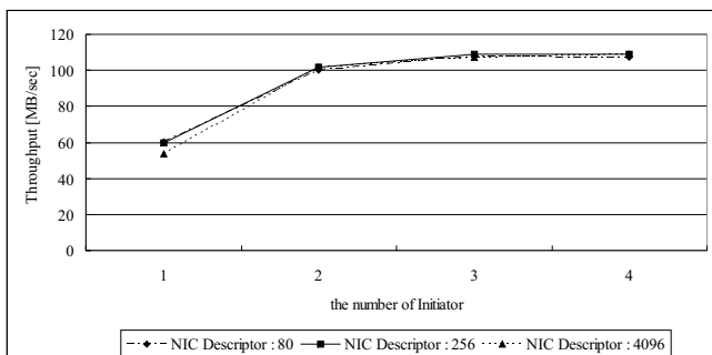
図 6 スループット測定結果
