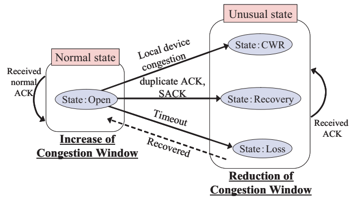
図1 Linux TCP 実装の状態遷移図
